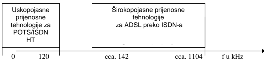
Slika 1. Frekvencijski opseg za uskopojasne i širokopolasne prijenosne tehnologije
