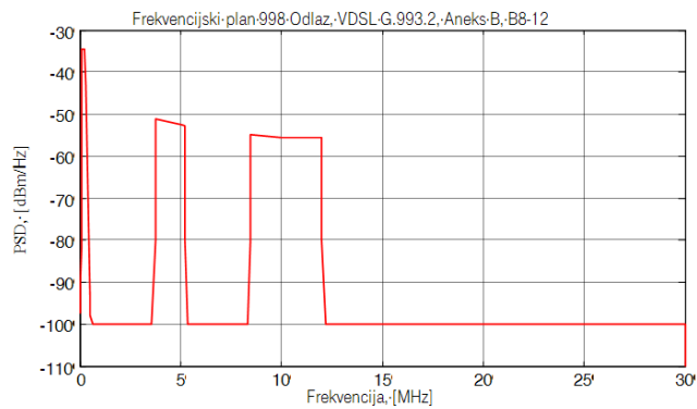
Slika 5.6.3 Frekvenijski predložak za odlazni smjer prijenosa za VDSL2, frekvenijski plan 998, B8-12
